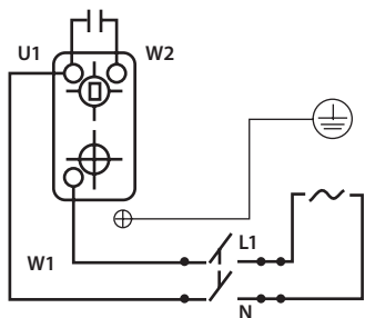
Diagrama eléctrico de instalación
